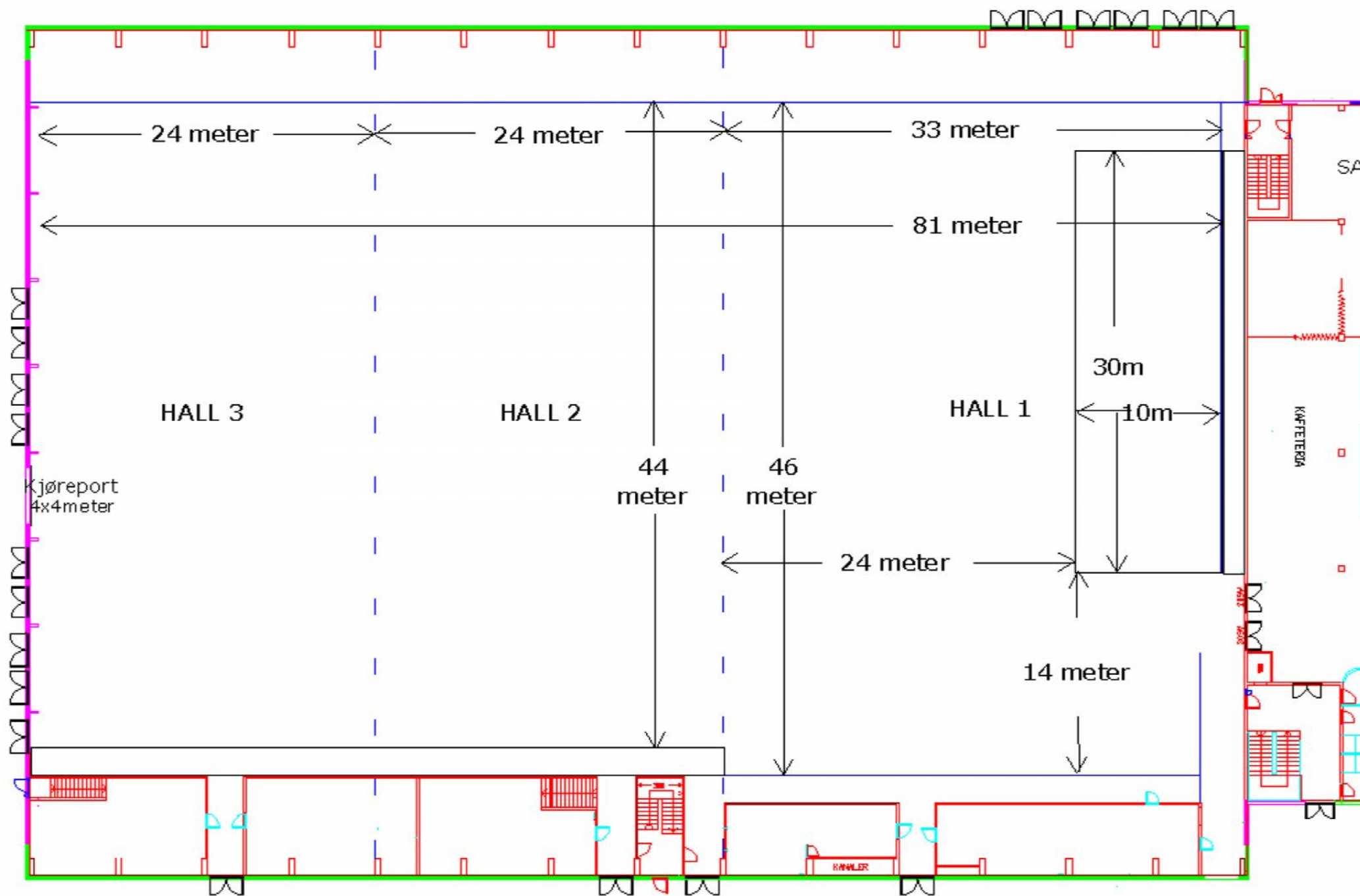
LETO HALLEN . PLAN 1 .
